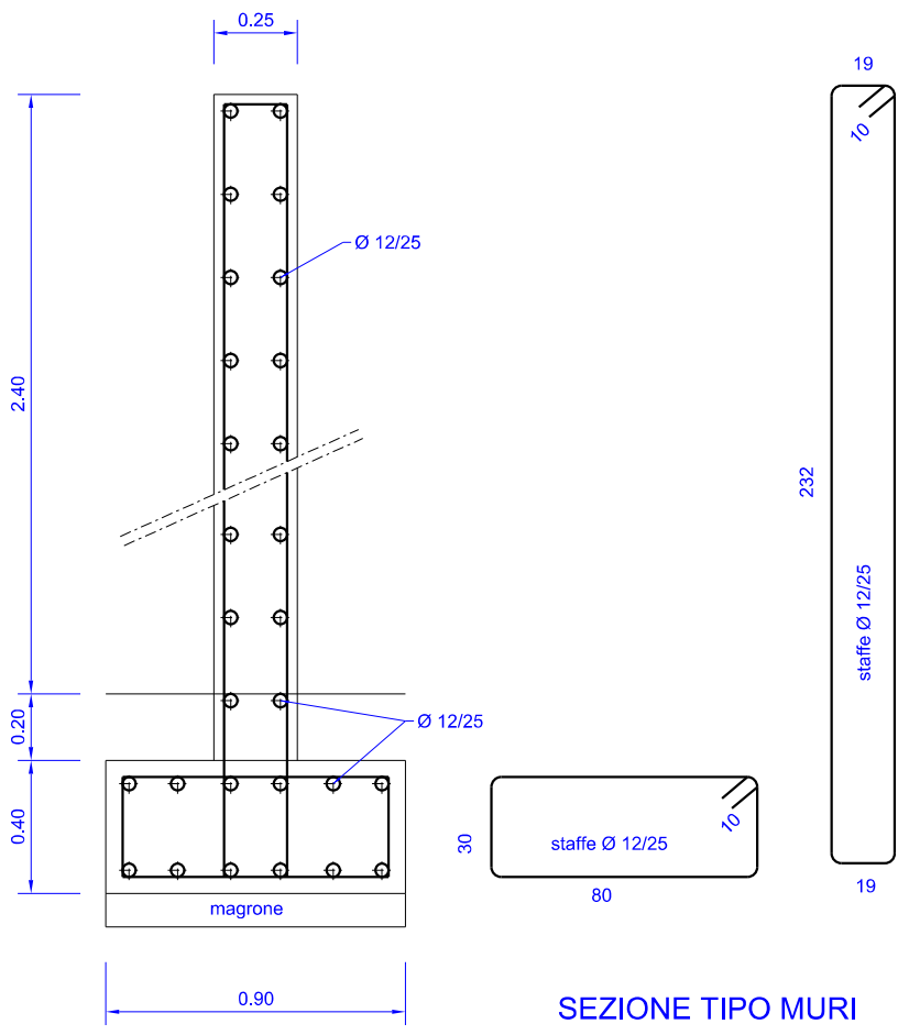
SEZIONE TIPO MURI
