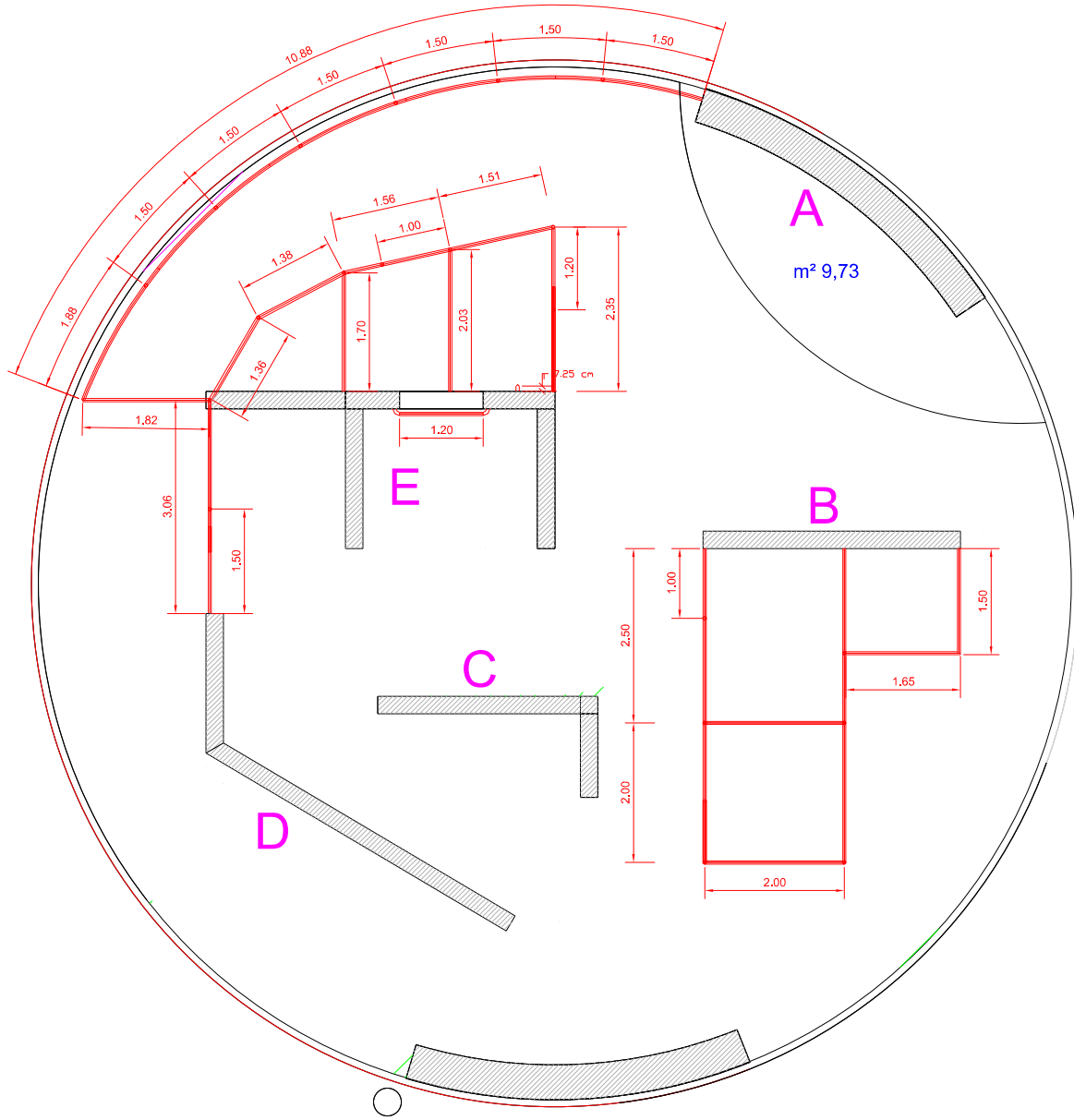
ZONA PARKOUR QUOTATURA TUBI
